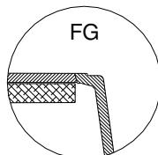
FG = 15° Flächenbündig
